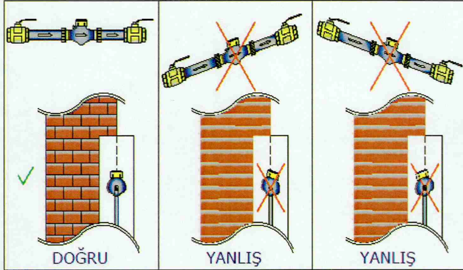
Şekil 1.1: Sayaçların Tesisata Bağlantısı
