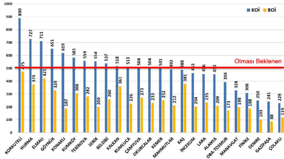
2022-ASAT ATIKSU ARITMA TESİSLERİ HAM ATIKSU KİRLİLİK KONSANTRASYONLARI-YILLIK ORT. mg/lt
