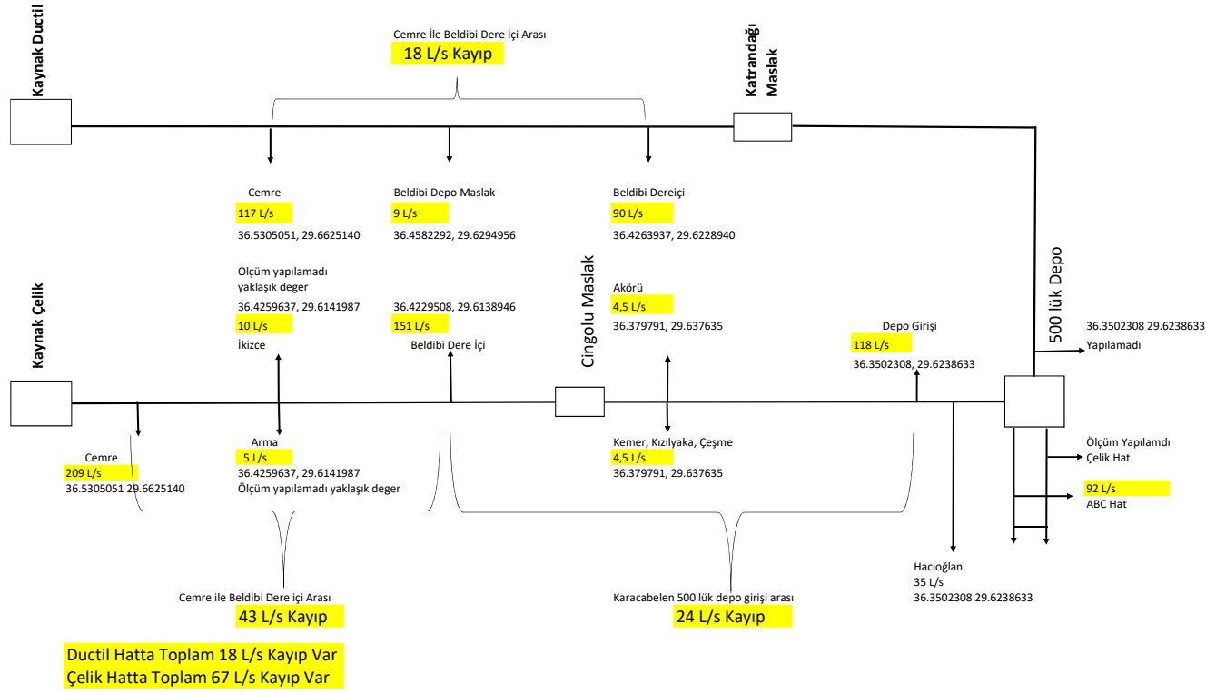
Gömbek Kaş hattı Fiziki kaçak Debi ölçüm çalışmaları
