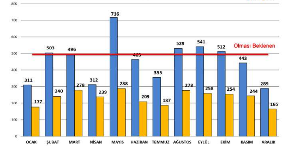
2022- LARA ATIKSU ARITMA TESİSİ HAM ATIKSU KOİ ve BOİ KONSANTRASYONLARI mg/lt
