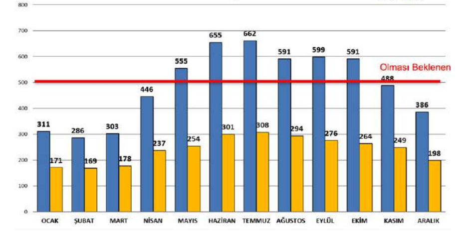
2022- İLÇE ATIKSU ARITMA TESİSLERİ (MERKEZ HARİÇ) HAM ATIKSU KİRLİLİK KONSANTRASYONLARI mg/lt
