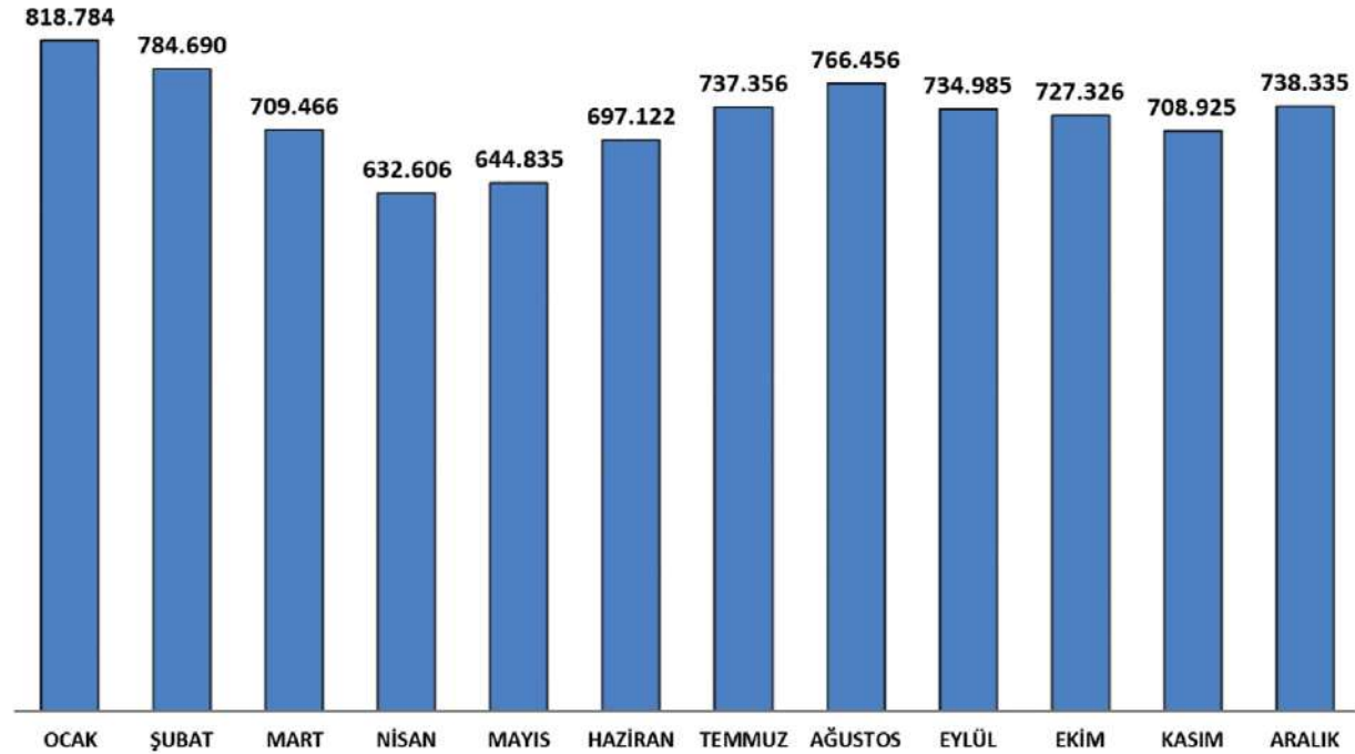
2022-ASAT ATIKSU ARITMA TESİSLERİ TOPLAM ATIKSU DEBİLERİ-AYLIK ORT. m 3 /gün
