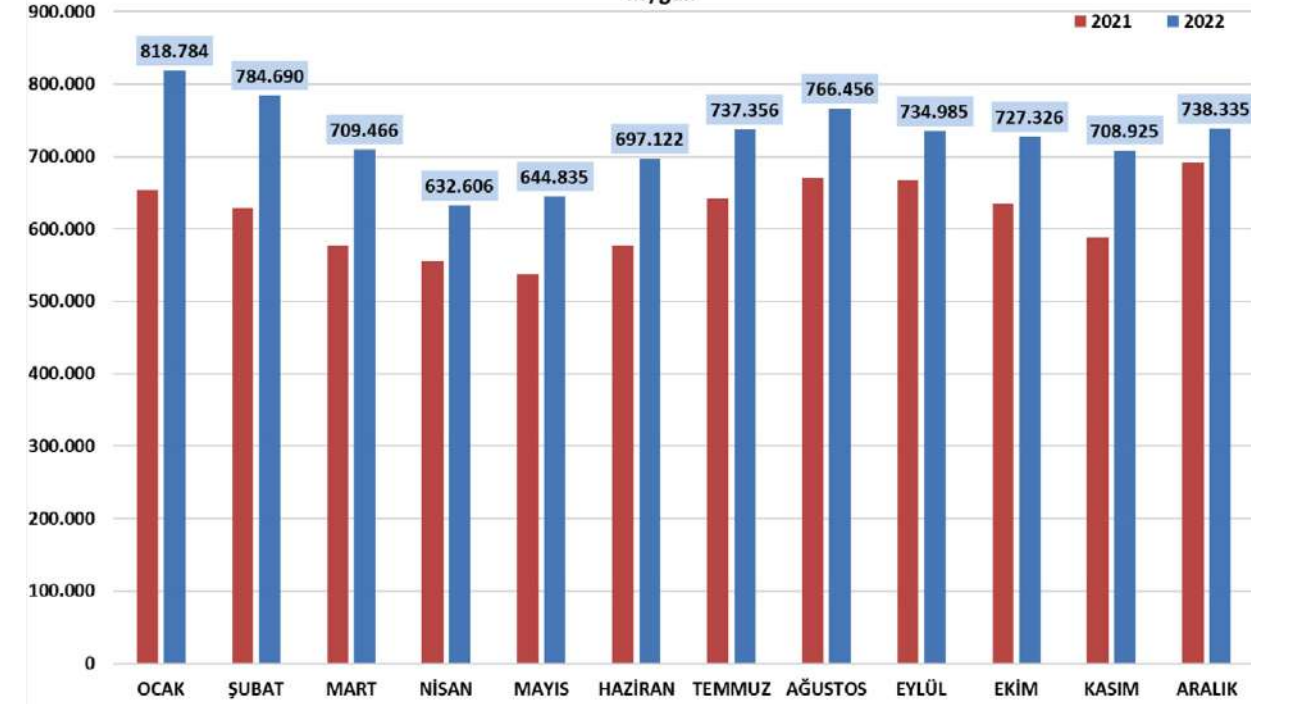
ASAT ATIKSU ARITMA TESİSLERİ TOPLAM ATIKSU DEBİLERİ-AYLIK ORT. m 3 /gün
