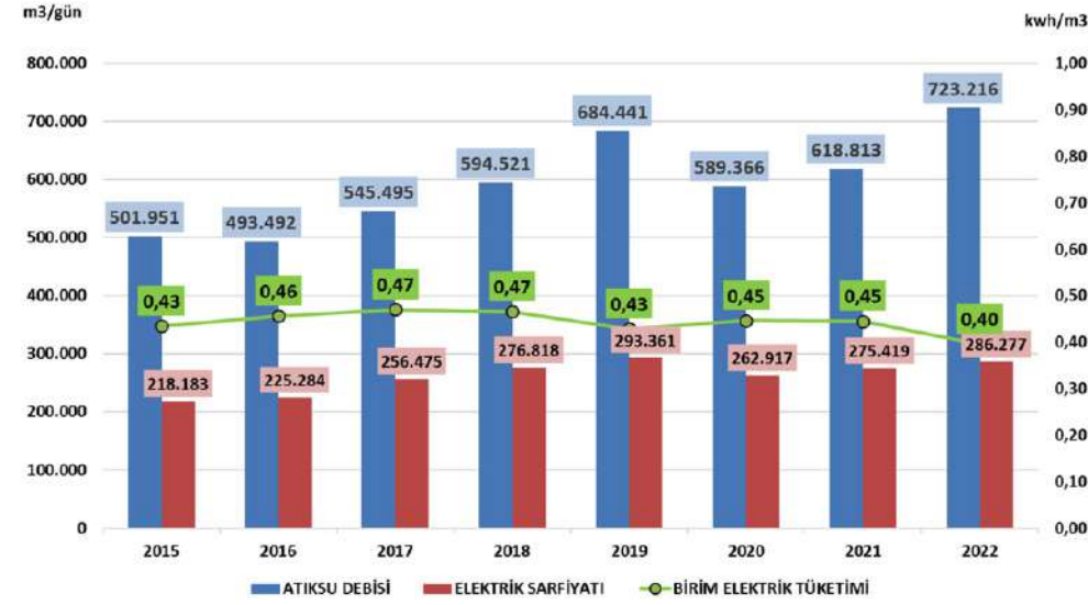
ASAT ATIKSU ARITMA TESİSLERİ ATIKSU DEBİSİ VE ELEKTRİK TÜKETİMLERİ m³/gün - kWh/gün
