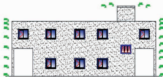
ARKA GÖRÜNÜŞ Ö: 1/10
