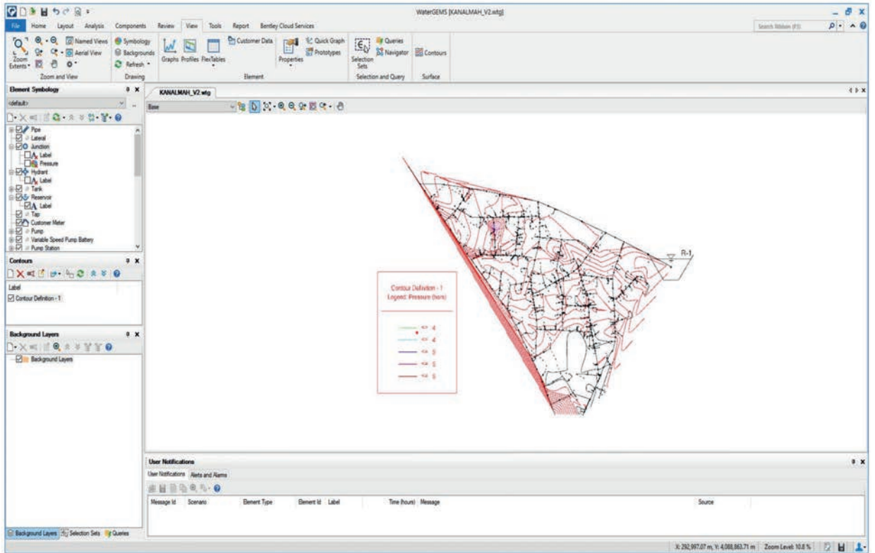
Kanal Mahallesi hidrolik model çalışması
